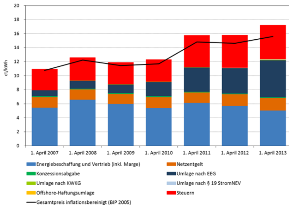
Abb. 11-3: Strompreise für nicht-begünstigte Gewerbe- und Industriekunden
