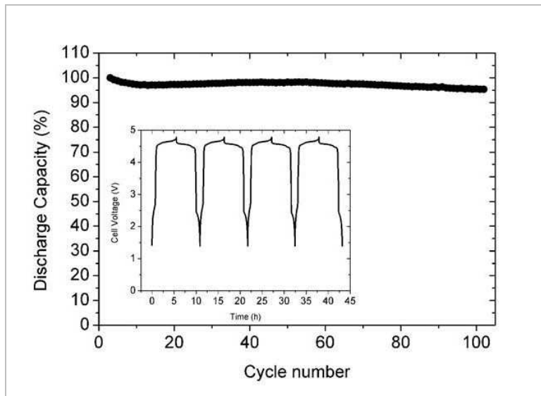
Zyklenstabilität einer Lithium-Ionenvollzelle mit neuem Kathodenmaterial; Lade/Entladeprofile der Zelle (insert). Grafik: ZSW
