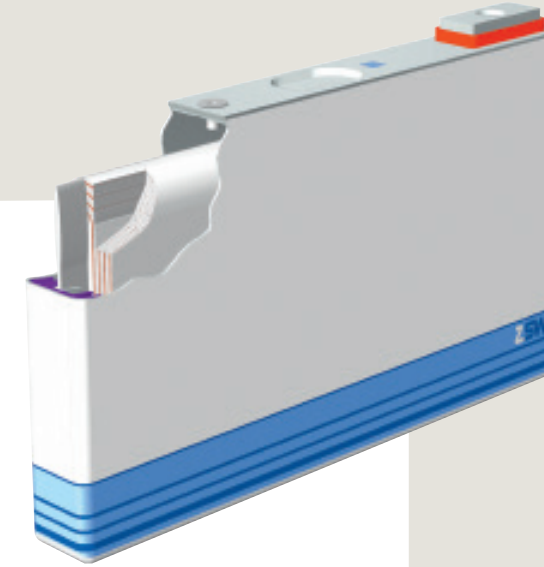
ZSW-Zelle nach DIN-Standard
